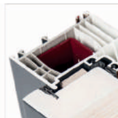
Six-chamber PVC door frame
